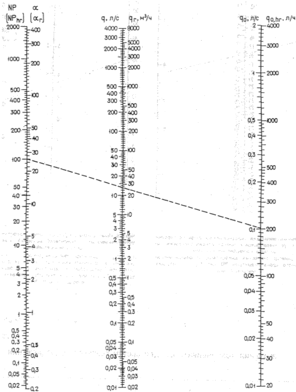
Черт.4. Номограмма для определения секундных и часовых расходов воды в зависимости от NP ( NP_{hr} ) при различных значениях q_0, \text{ л/с} , q_{0,hr}, \text{ л/ч}
